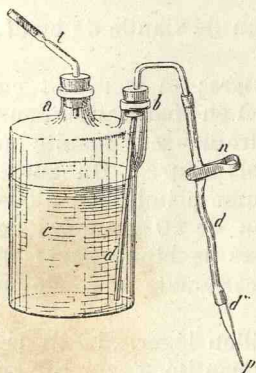
Fig. 19. — Conserve de bouillon.
