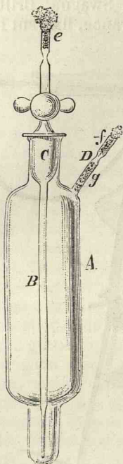
Fig. 29. — Appareil de Straus et Wurtz pour compter les germes de l'air en faisant barboter ce dernier dans la gélatine. — A, tube dans lequel est enfermée la gélatine; e, C, B, bouchon tubulé qui donne accès à l'air chargé de germes; D, tube d'aspiration.
