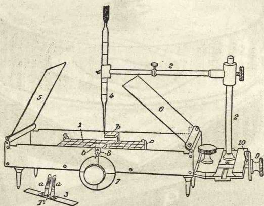
Fig. 32. — Analyseur bactériologique d'Arloing. — 1, plaque porte-gélatine; 2, 2, porte-pipette; 3, couvre-joints isolé; 4, pipette; 5, 6, couvercles en verre de l'analyseur; 7, bouton moteur de la crémaillère qui déplace la plaque de gélatine; 8, repère; 9, bouton moteur de la crémaillère qui déplace le porte-pipette; 10, repère. — Le couvre-joints 3 est isolé : T, orifice dans lequel s'engage l'extrémité capillaire de la pipette; a, a, languettes ressorts entre lesquelles passe la pipette; b, b, équerres métalliques sur lesquelles glisse le couvre-joints.
